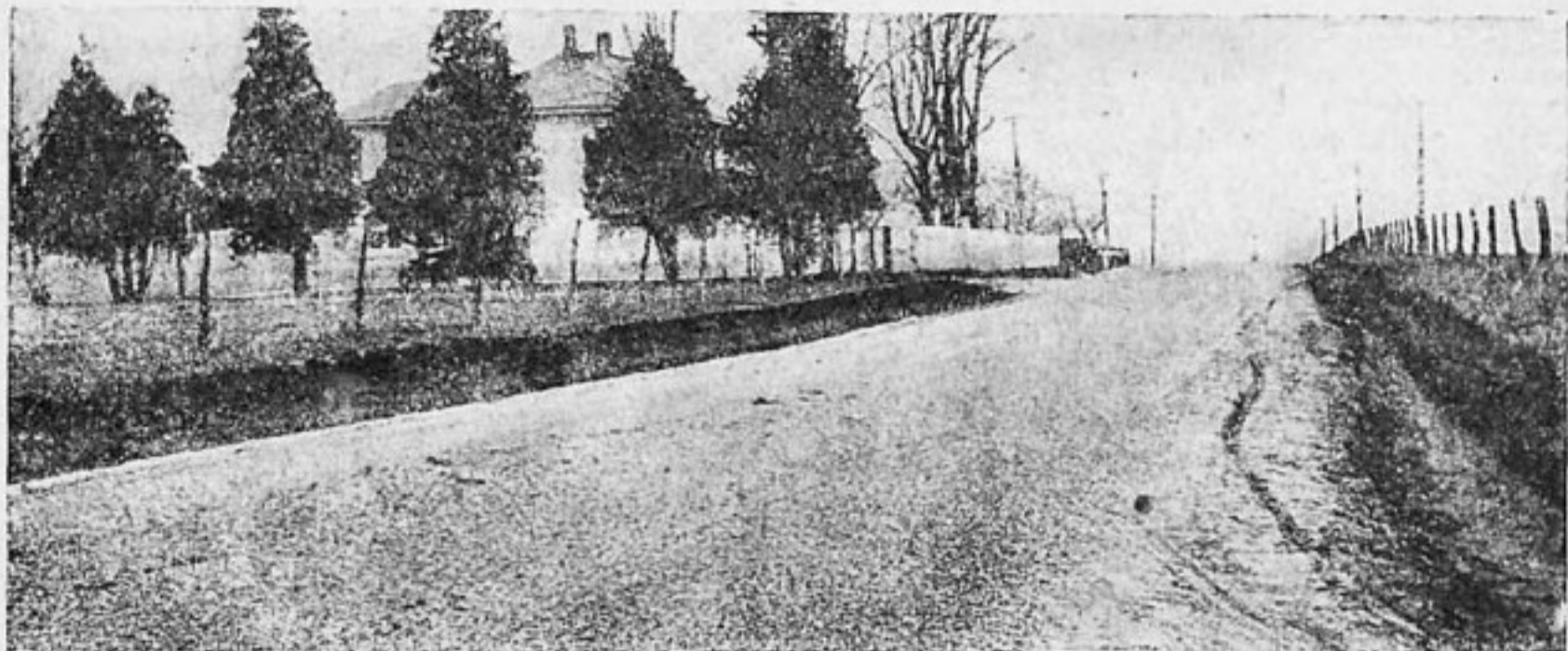
Гравийная дорога, построенная без применения катков. Уплотнение достигалось проездом при помощи стругов и утюгов с постепенным наращиванием коры из валов гравия, заготовленных по сторонам дороги.
